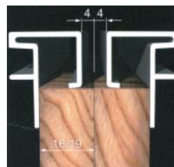
Kein Fräsen im Schrank Völlig Vorsetzsystem. Pas de fraisage dans les côtés. Système complet à monter sur l'armoire.
